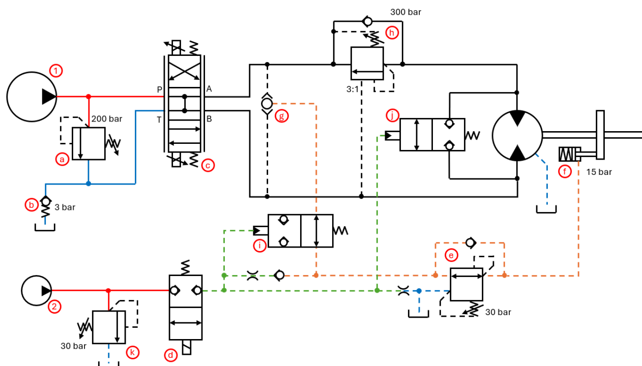
Schéma d'un circuit hydraulique de treuil (présenté lors de la partie 1).
