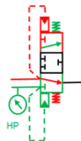
AVEC LA HP SUR LA LIGNE ROUGE (FUITE SUR LA LIGNE ROUGE)
