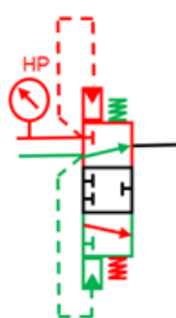
AVEC LA HP SUR LA LIGNE ROUGE (FUITE SUR LA BP VERTE)
