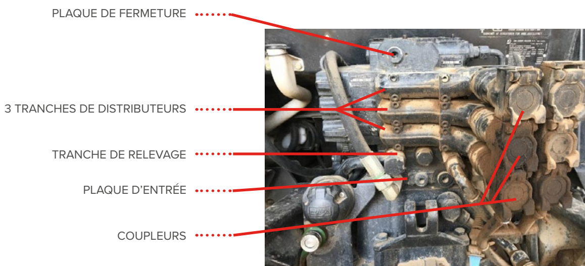
Pack arrière avec fonderie pour coupleurs
