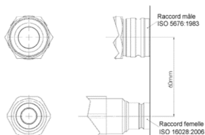
CONNECTION DES 2 CONDUITES DE FREINAGE HYDRAULIQUES.
